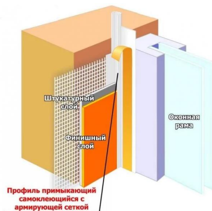
Рис.24. Профиль примыкающий с армирующей сеткой
